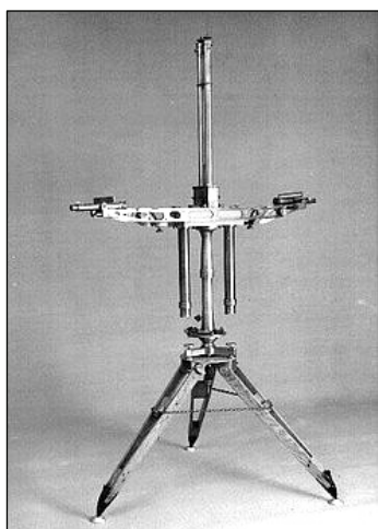
Torziós inga
